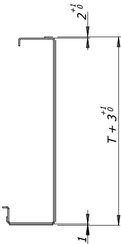
DOOR HEADER
