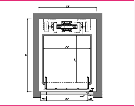
KABINENFALTTÜR, SCHACHTDREHTÜR
