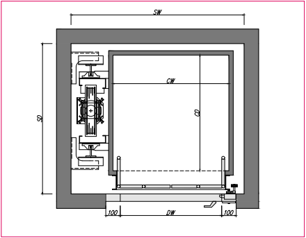
KABINENFALTTÜR, SCHACHTDREHTÜR
